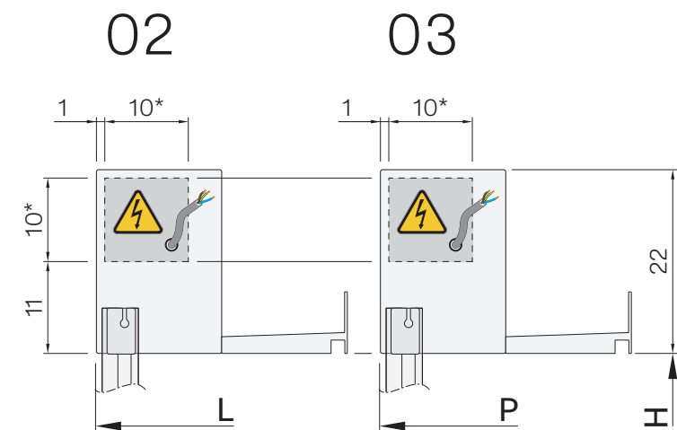
FISSAGGIO A MURO (Profilo Portante Esterno) WALL MOUNTING (External Supporting Profile) FIXATION MURALE (Profilé Porteur Externe) WANDBEFESTIGUNG (Äußeres Tragprofil)
