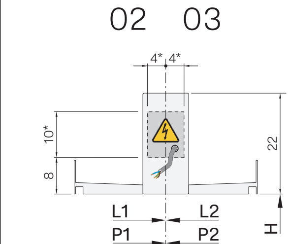
FISSAGGIO A MURO (Profilo Portante Intermedio) WALL MOUNTING (Intermediate Supporting Profile) FIXATION MURALE (Profilé Porteur Intermédiaire) WANDBEFESTIGUNG (Mittleres Tragprofil)
